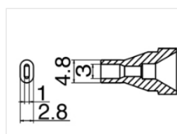
N61-15 Düse
