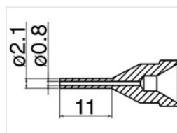
N61-11 Düse
