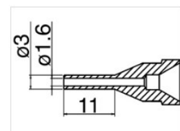
N61-14 Düse
