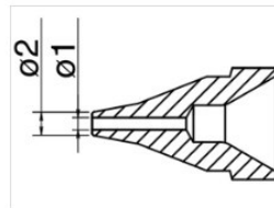
Düse N61-05
