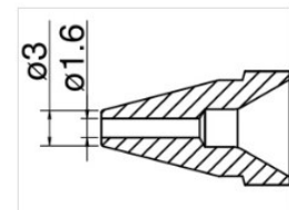
N61-10 Düse
