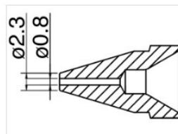
Düse N61-07
