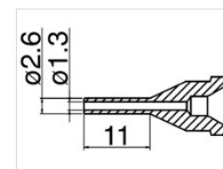
N61-13 Düse
