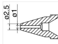
Düse N61-08
