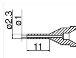
N61-12 Düse
