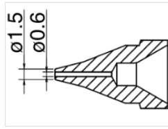
Düse N61-01
