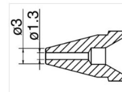
Düse N61-09
