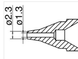
Düse N61-06
