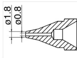
Düse N61-04
