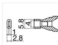
N61-16 Düse
