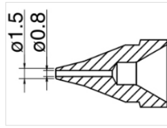
Düse N61-02
