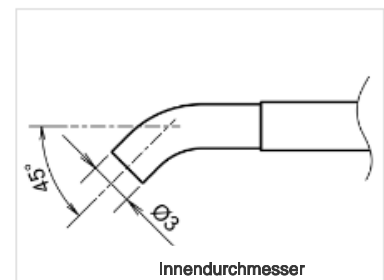
NA01-CB30 Düse
