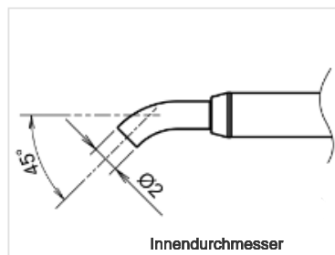
NA01-CB20 Düse
