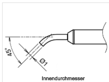
NA01-CB10 Düse
