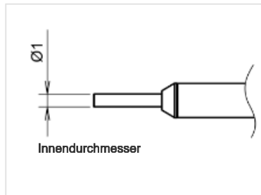
NA01-C10 Düse
